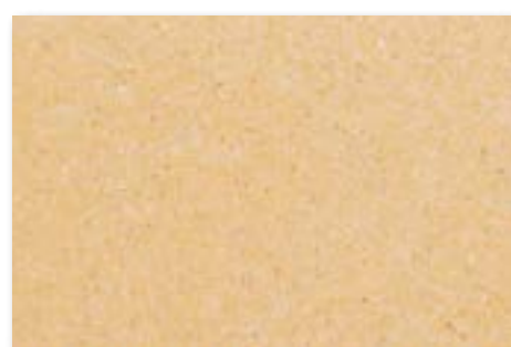
AMARELO NEGRAIS MDJ1020114 NEGRAIS YELLOW 58x38x2,5 cm / 58x58x2,5 cm ≈ 62 Kg/m 2
