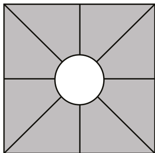
BD1 BASE DE DUCHE DE PISCINA POOL SHOWER BASE Ø 20 / 30 cm 120x120x2,5 cm ≈ 82 kg/Un
